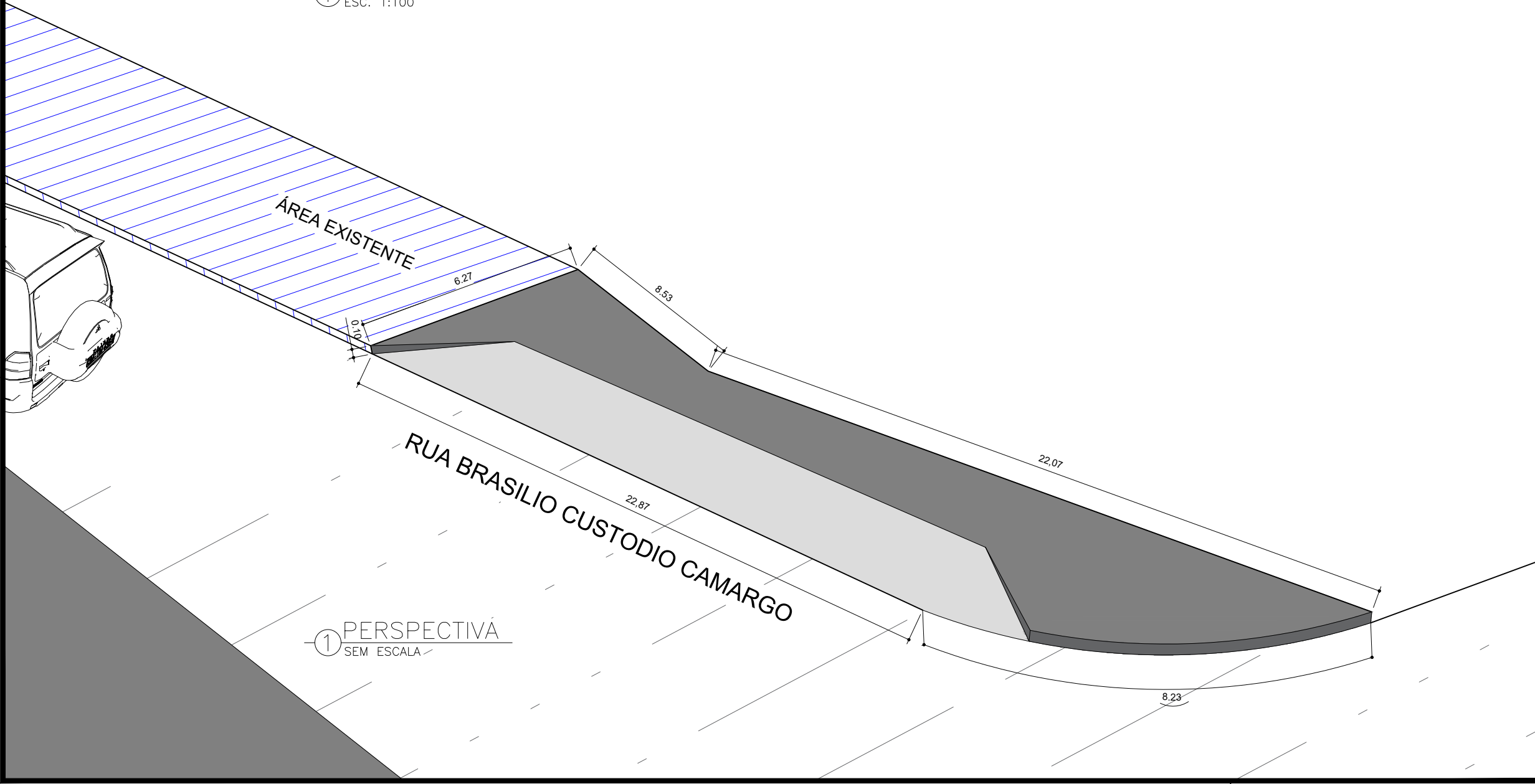
① PLANTA BAIXA ESC. 1:100
